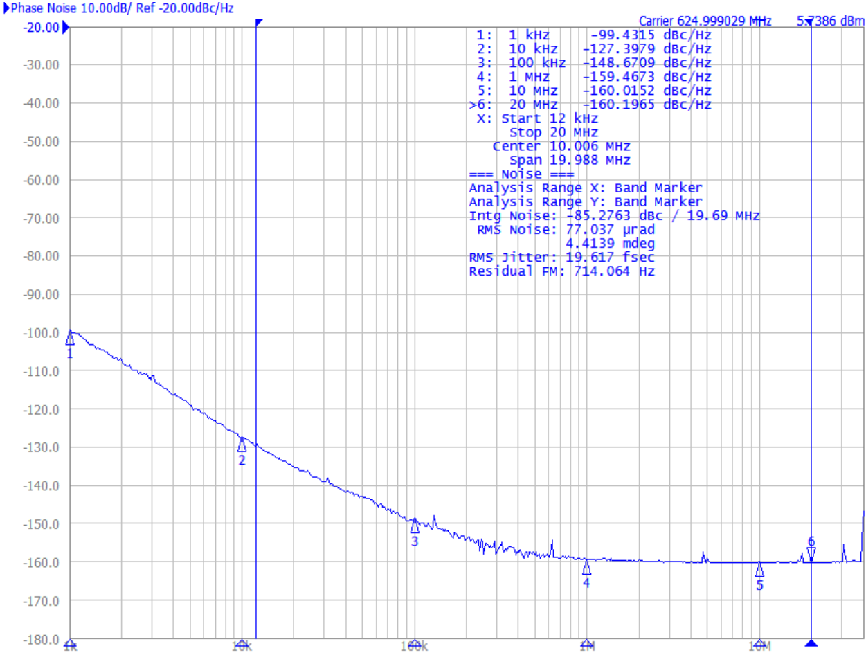
Figure 5. Carrier: 625 MHz
