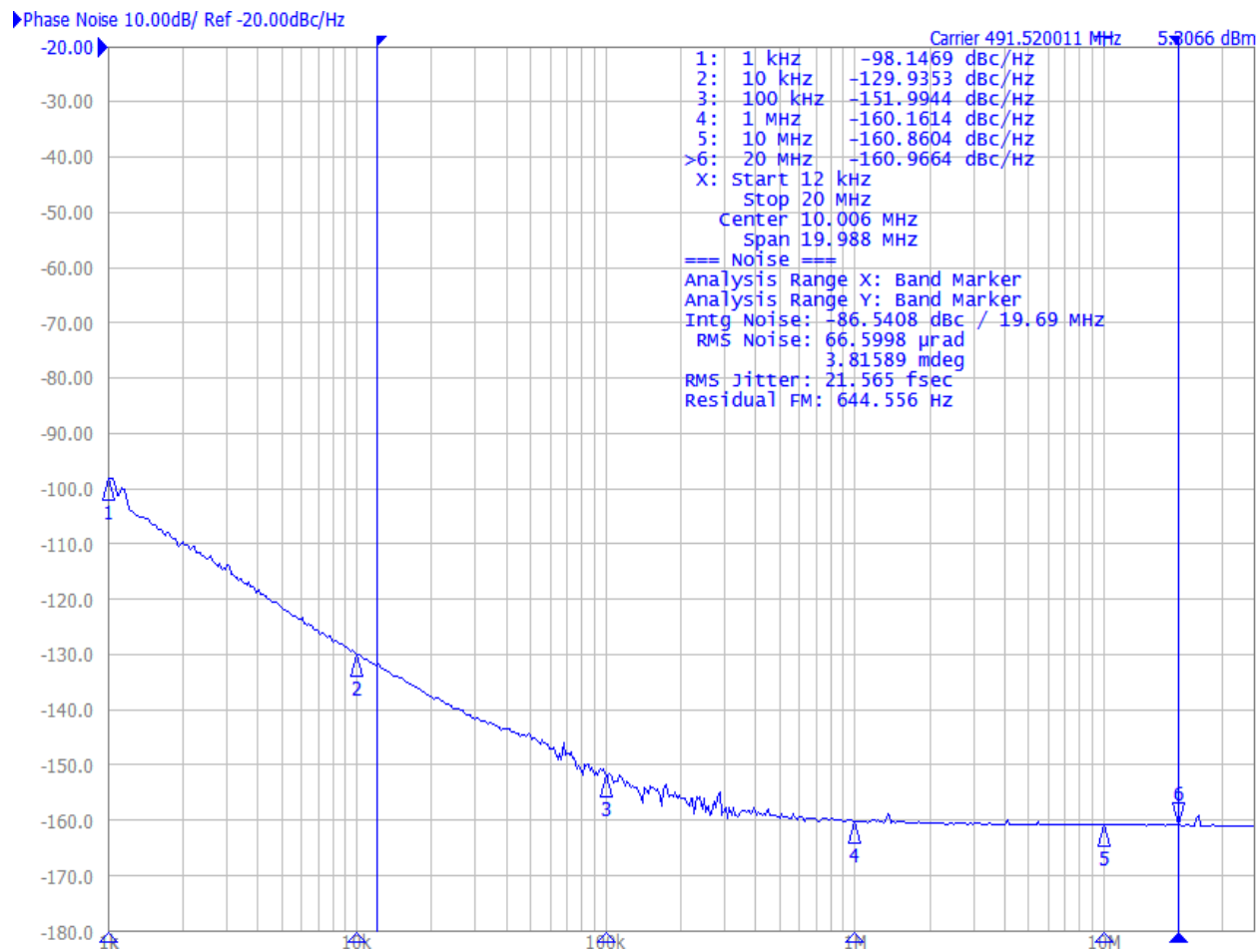
Figure 6. Carrier: 491.52 MHz
