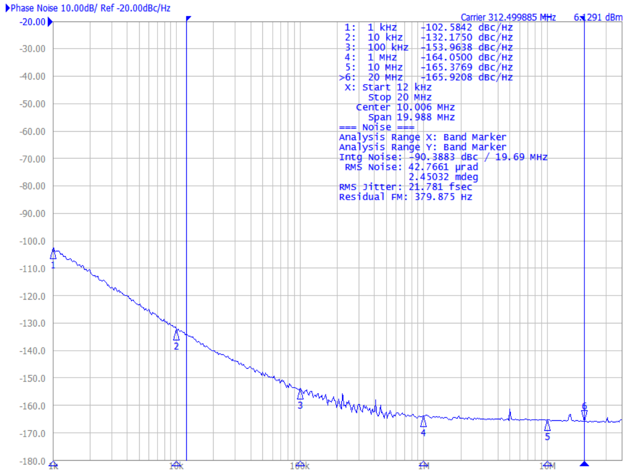
Figure 7. Carrier: 312.5 MHz
